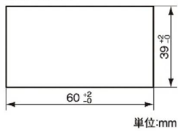
取付寸法図
