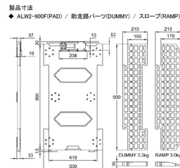
画像は、PADの寸法図です。
