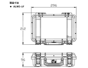
画像は、指示計：データBOXの寸法図です。
