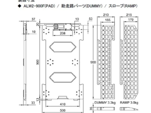
画像は、PADの寸法図です。
