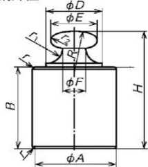
分銅外径図
